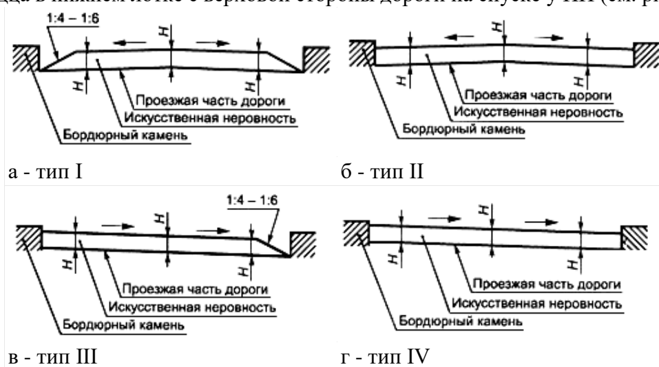
Рисунок 2 - Продольные профили ИН
