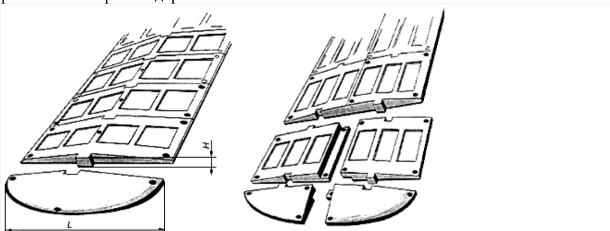
а - ИН из одной части основного и краевого элементов
