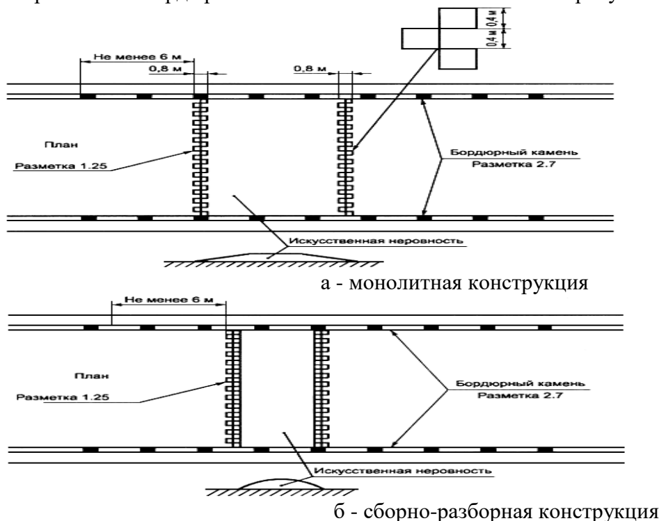
Рисунок 4 - Пример нанесения разметки 1.25 и 2.7 при устройстве ИН
